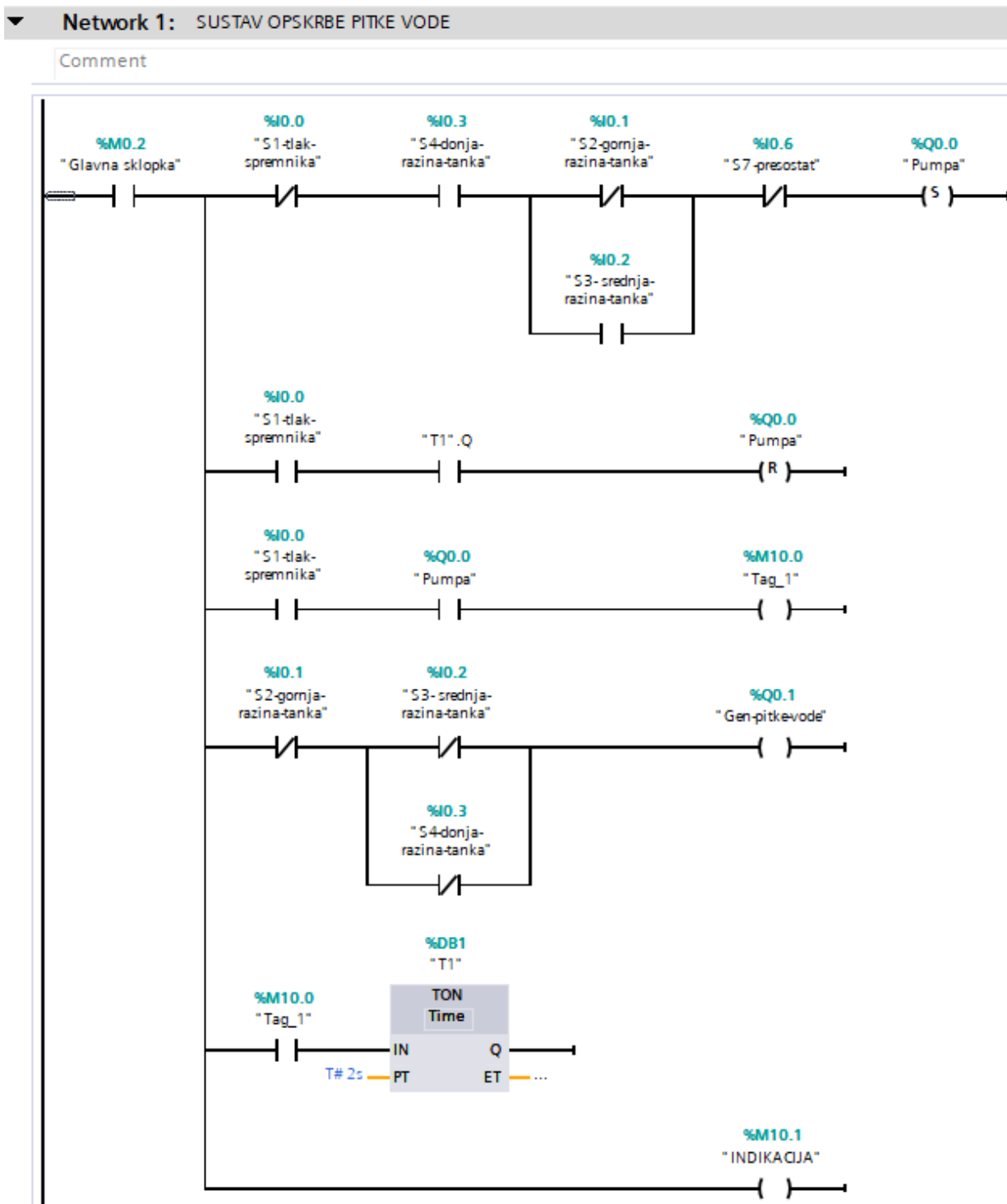
Slika 47. Dijagram sustava
