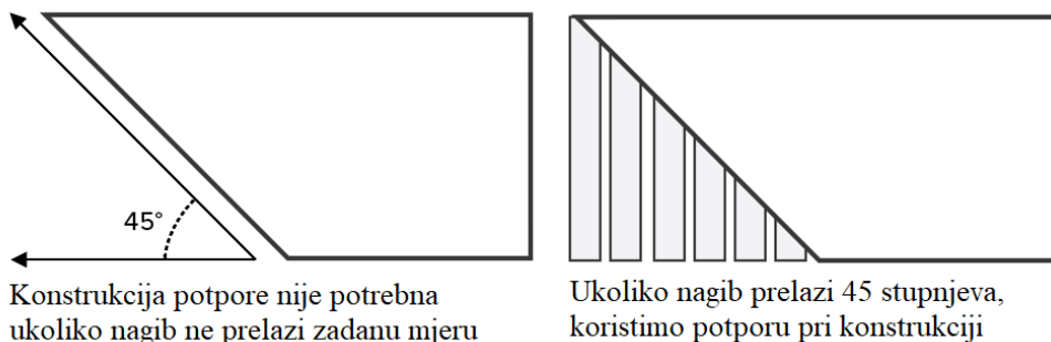
Slika 42. Konstrukcija potpore [10]
