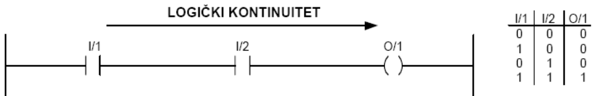
Slika 3.2. Logička operacija 'I' [4]
