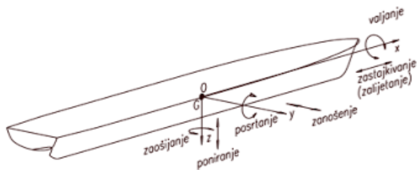
Slika 22. Prikaz translacijskih i rotacijskih pomaka broda [7]
