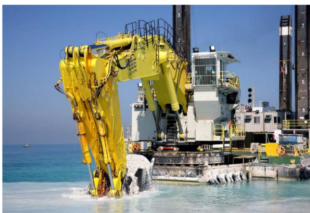
Slika 28. Backacter 1100, najveće jaružalo s dubinskom lopatom, sa sustavom elektroničkog pozicioniranja [27]
