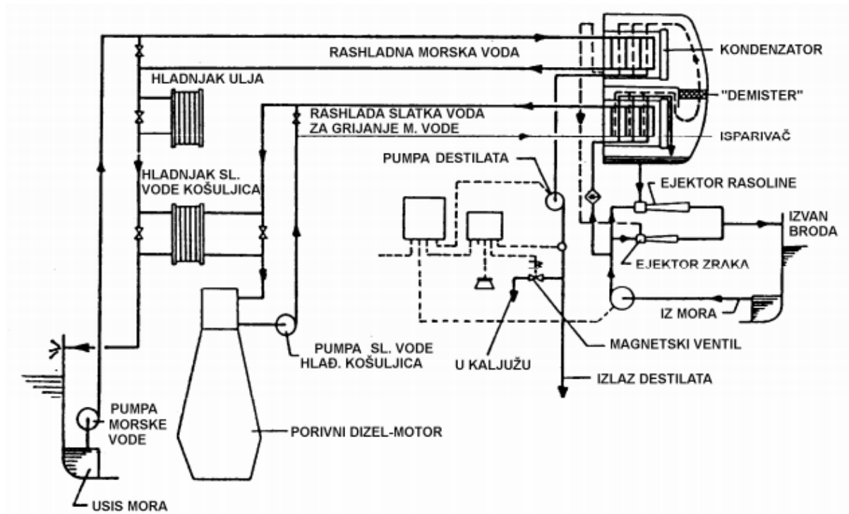
Slika 4. Shematski prikaz vakuumnog evaporatora [3]
