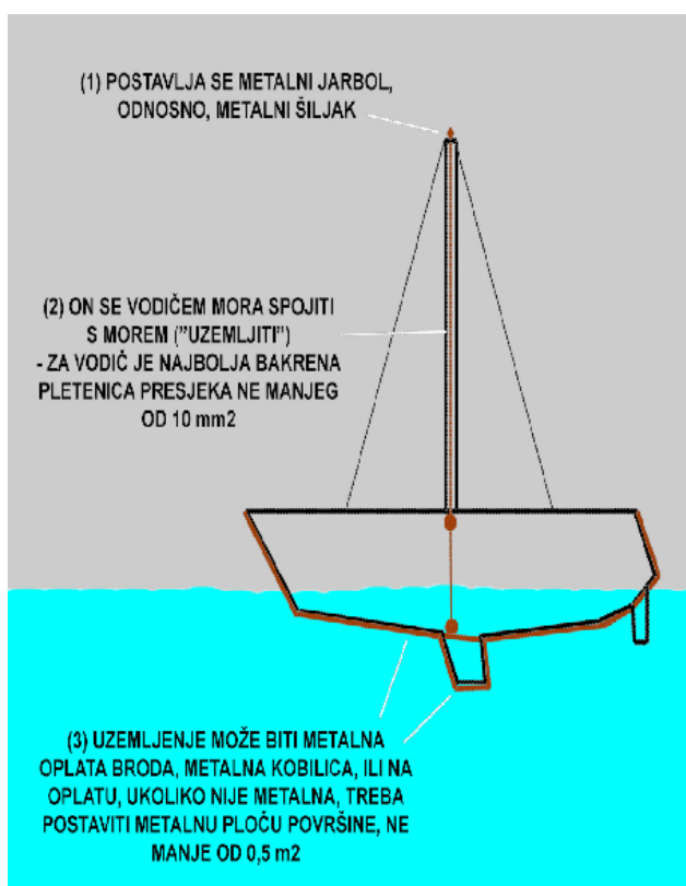
Slika 7. Gromobranska zaštita
