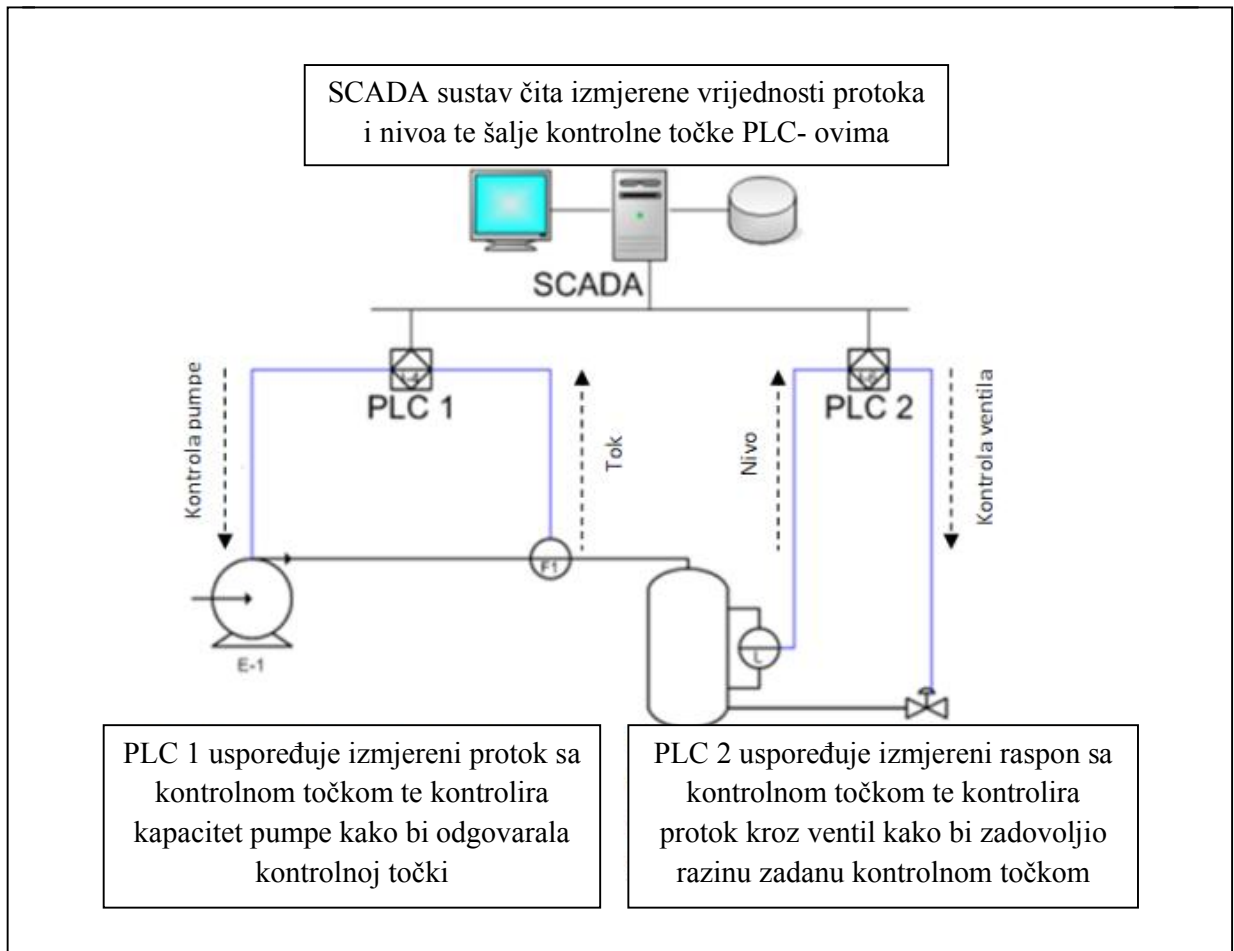
Slika 24. Shematski prikaz sustava za nadzor razine [15]
