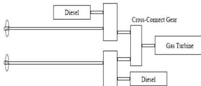
Slika 2. CODAG postrojenje[10]
