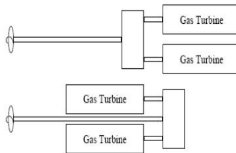
Slika 1. COGAG postrojenje[10]
