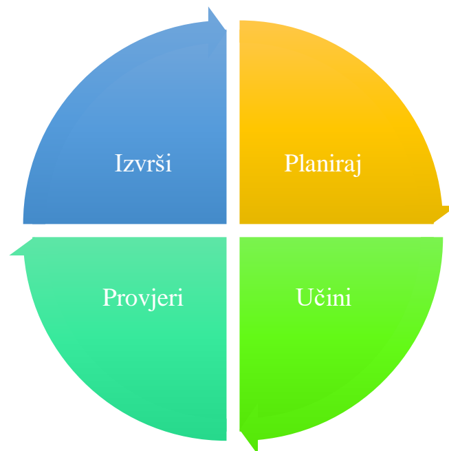
Slika 8. PDCA ciklus [32]
