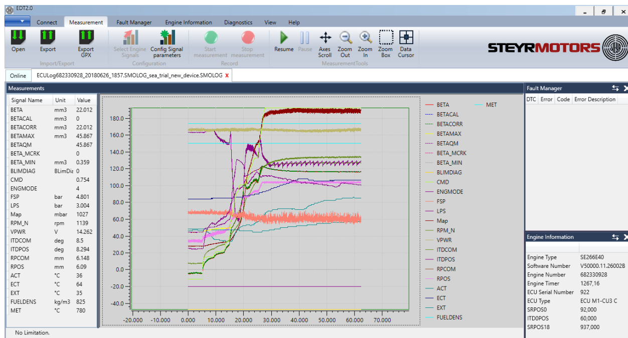
Slika 35. Prikaz snimljenih parametara motora [8]
