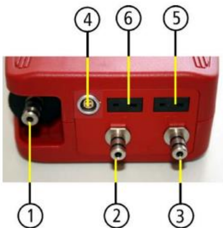
Slika 11. Priključci Optima 7 NDIR mjernog uređaja [16]
