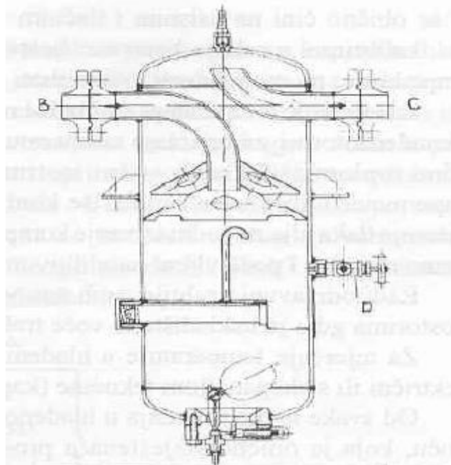
Slika 22. Odvajač ulja [11]
