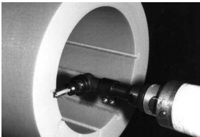
Slika 20. Glodanje utora [10]
