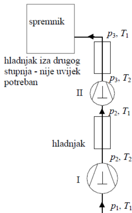
Slika 10. Dvostupanjska kompresija
